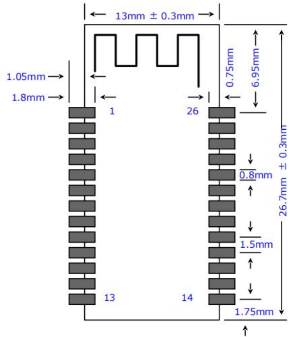
PCB 封装图
