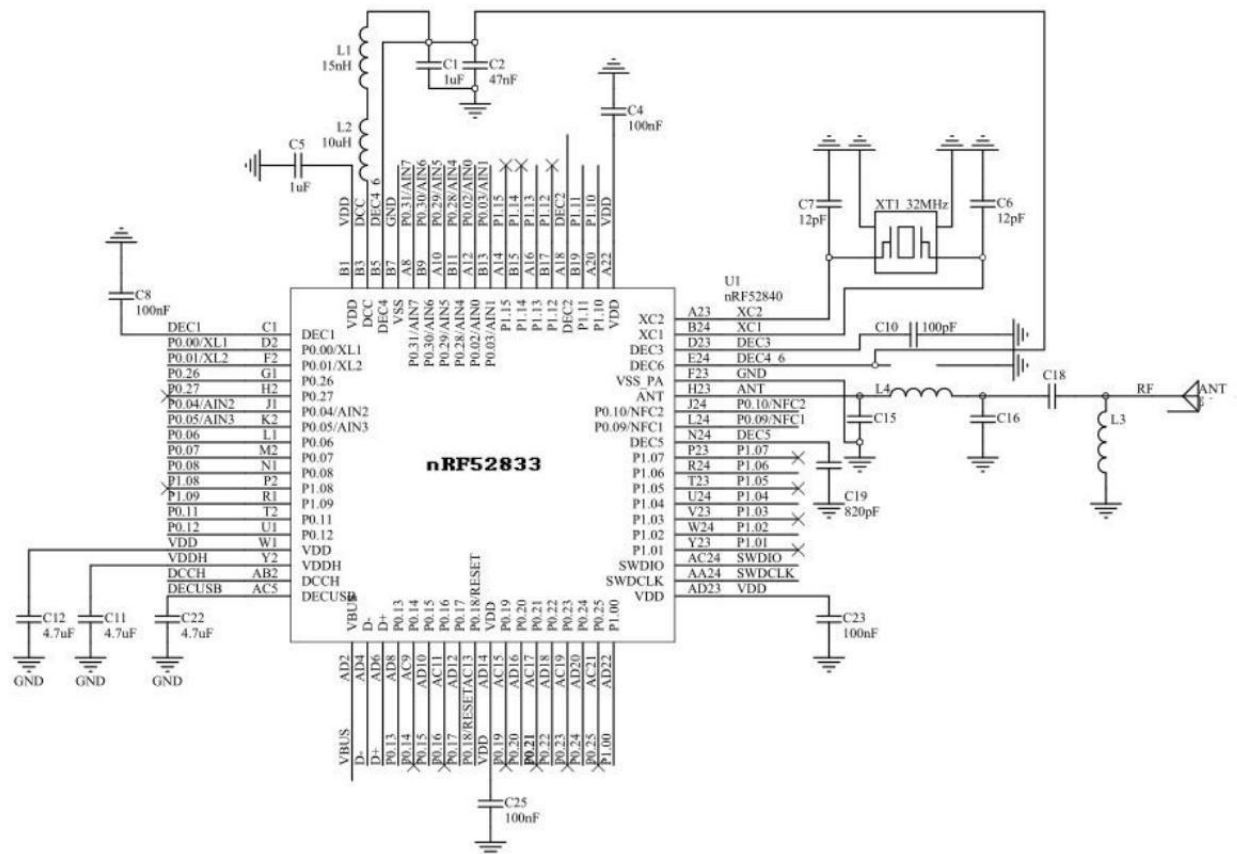
图 5-1 电路图
